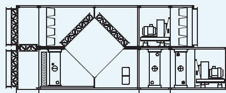
схема АКВ-5
