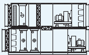
схема АКВ-2
