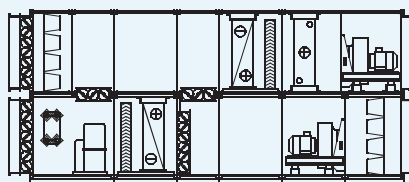
схема АКВ-4
