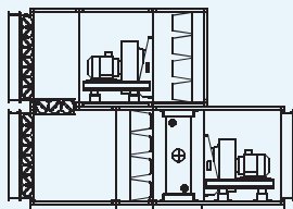
схема АКВ-1
